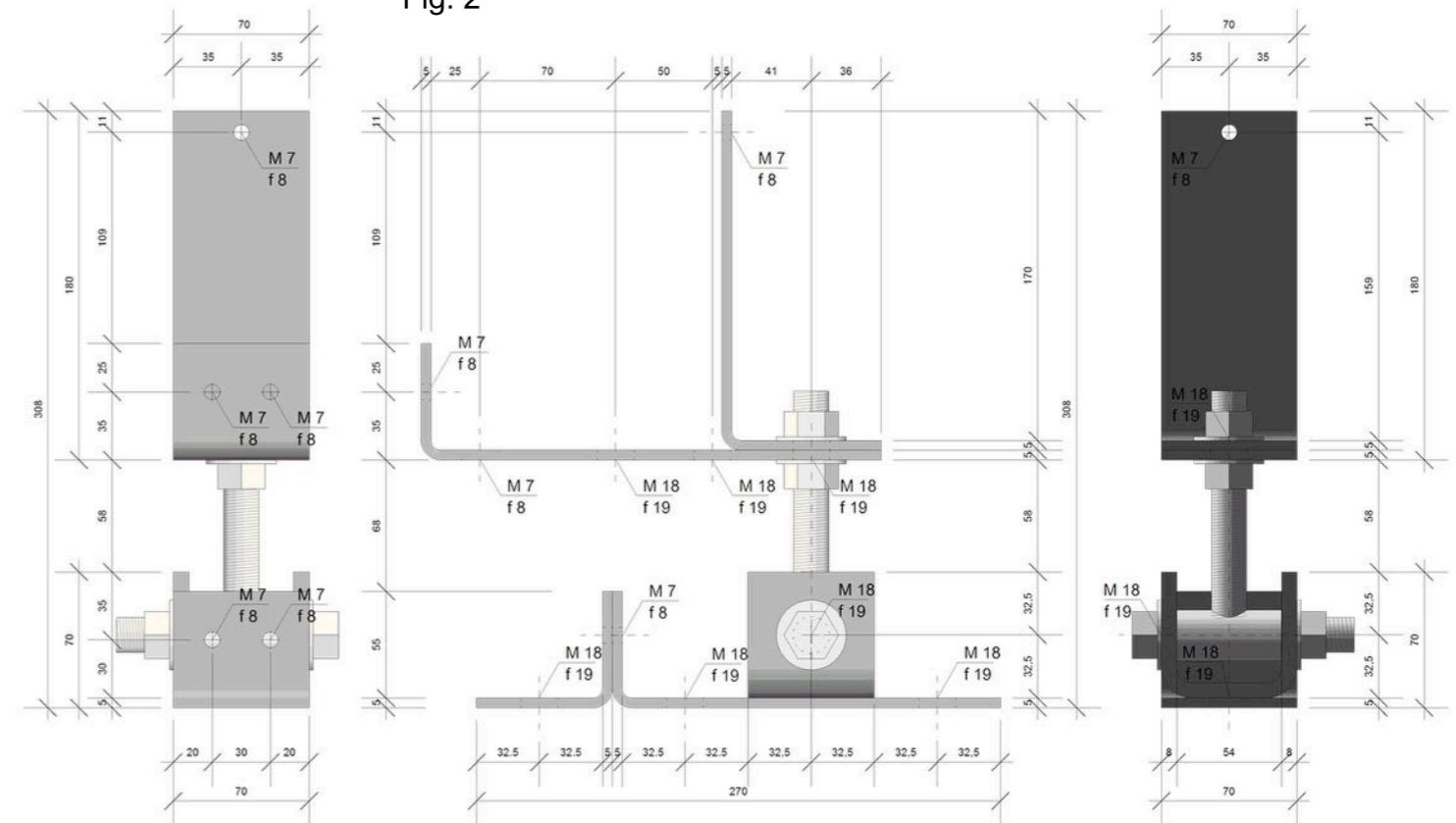
Fig. 3 Sez. 2-2
