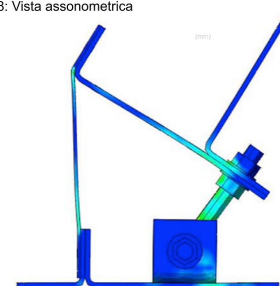
Fig. 9: Vista frontale
